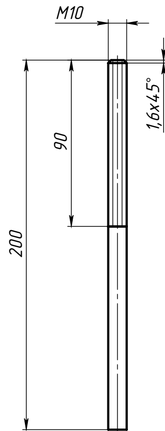
Поз.1 (Шпилька)
