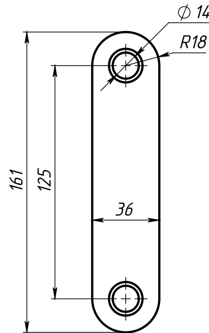
Поз.4 (Серьга)
