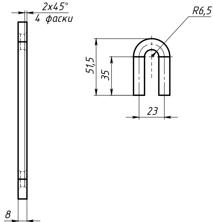
Поз.2 (Ушко)
