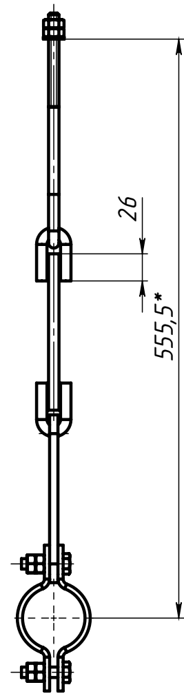
Поз.5 (Полухомут)
